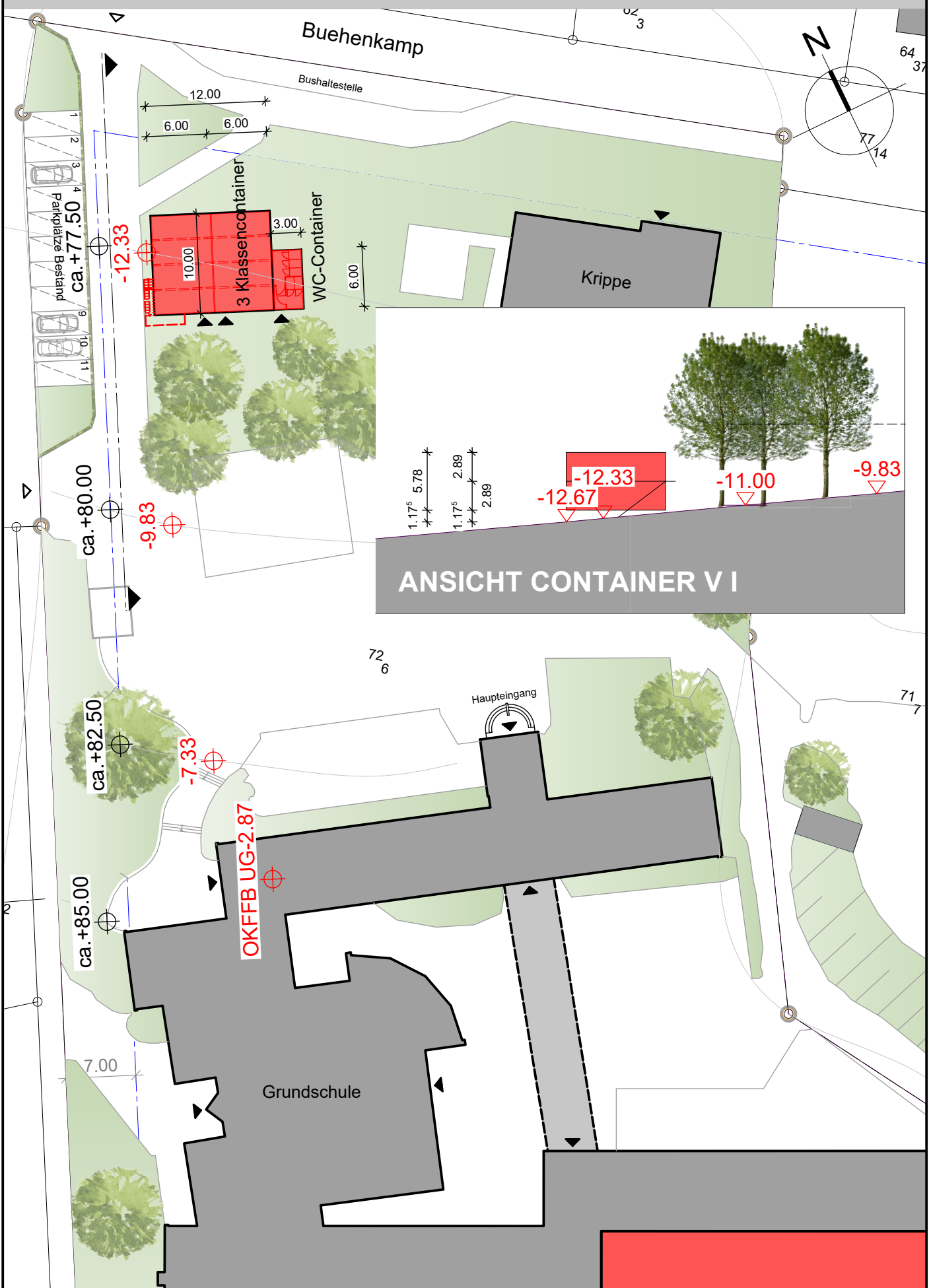
LAGEPLAN CONTAINER V I M. 1:500
